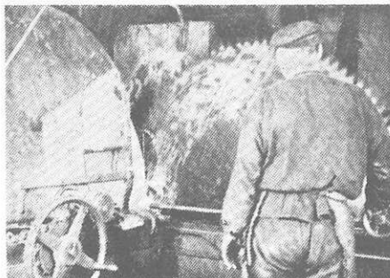
Slipning av cirkelsågar.
