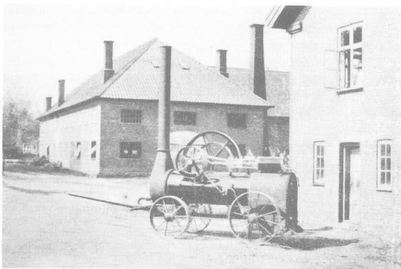
Transportabel lokomobil utanför de äldsta verkstäderna.
