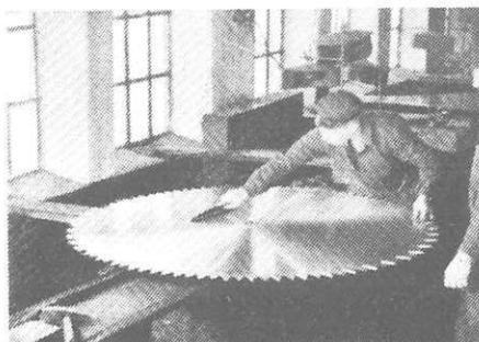
Riktning av cirkelsågar.
